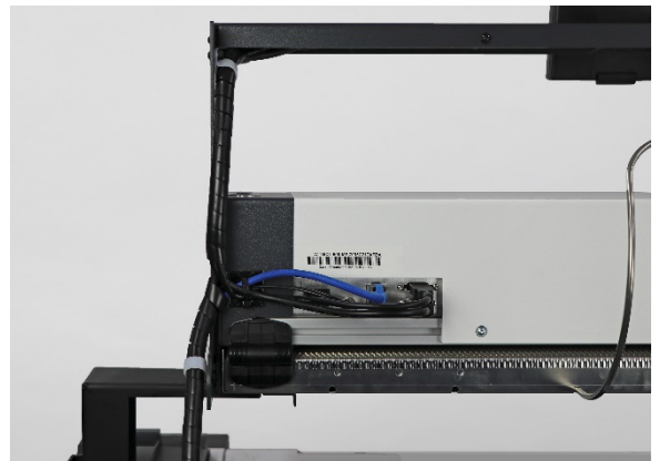
Rückansicht der Stecker und Kabelführungen
